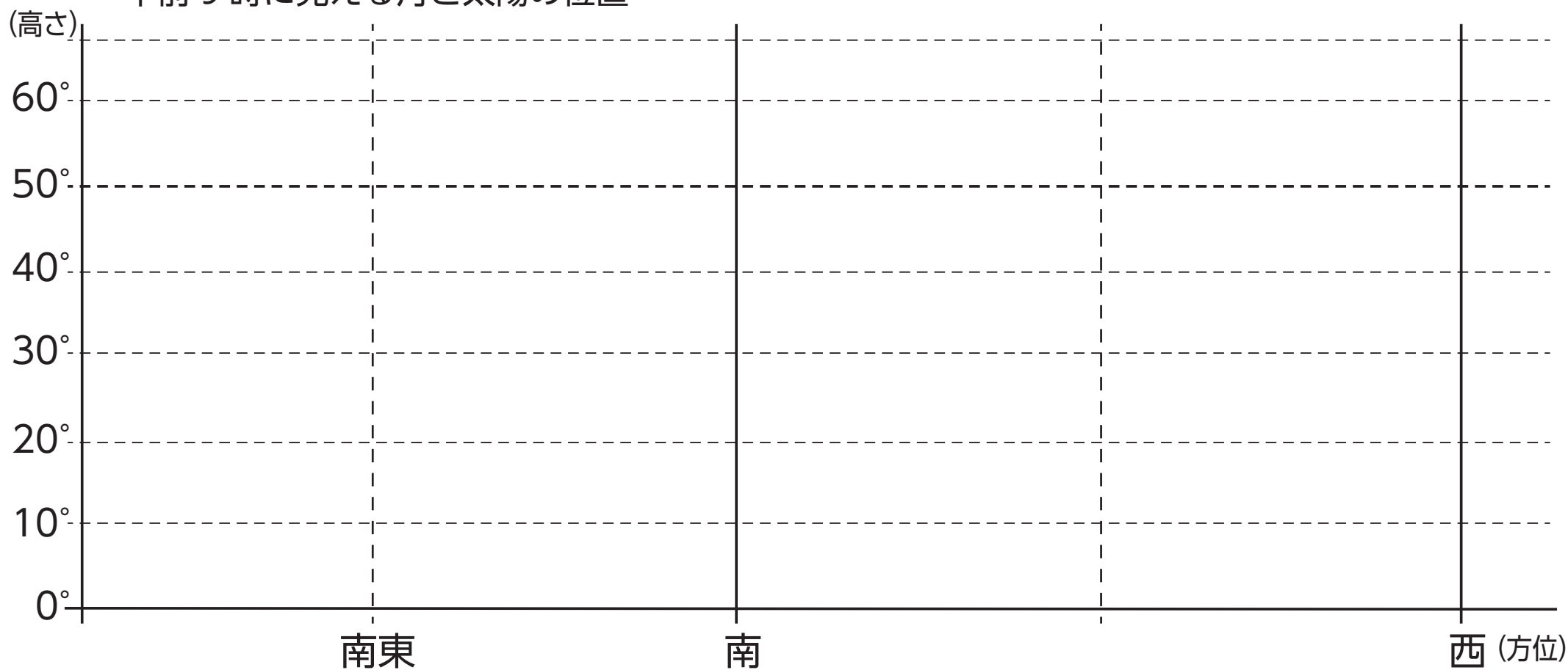
午前 9 時に見える月と太陽の位置
